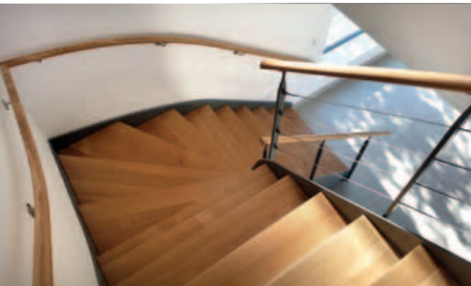
↗ Ma-1 : Escalier à structure métallique dite limon à la « française » thermolaqué, marches et mains courantes en chêne, poteau plat métal et câbles inox (norme PMR).
