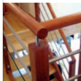
Ri-6 ➔ Détail assemblage des mains courantes sur poteau d'angle.
