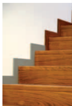
↔ Ma-5 → Escalier ERP métallique avec limon design découpe dessus dessous, rampe et main courante murale avec débord, bande antidérapante, nez de marche sans débord.
