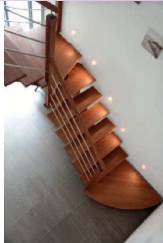
↗ Eq-5 → Escalier 2/4 tournant, en sapelli, marche de départ S7, poteau T6, main courante ronde. Deux positionnements des doubles crémaillères possibles.
